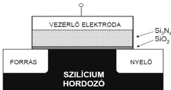
2. ábra Az MNOS memóriatranzisztor
