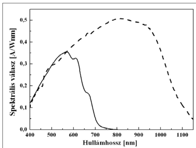
2. ábra Beltéri napelemek spektrális válasz ábrája: PIII cella (szaggatott) és referencia a-Si cella (folytonos). A spektrális válasz: egy optikai érzékelő reakciója, mértéke az érzékelő válaszában (generált áram) és az egységnyi hullámhossz-tartományban besugárzott teljesítménynek a hányadosa.
