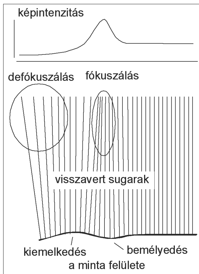
1. ábra A Makyoh-topográfia képalkotásának vázlata
