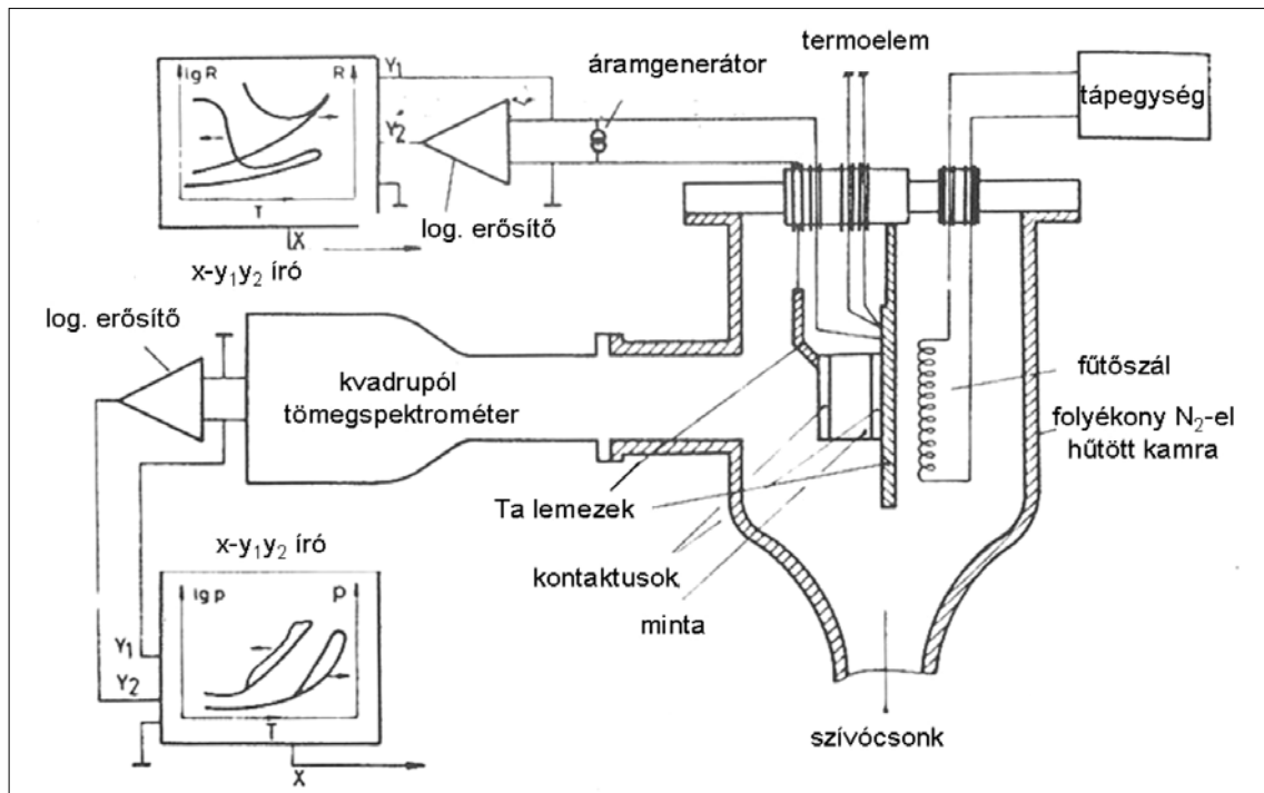
1. ábra Illékony komponens mérésére alkalmas kisnyomású kamra vázlata.
