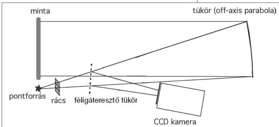
5. ábra Tükör alapú Makyoh-topográfias rendszer vázlata
