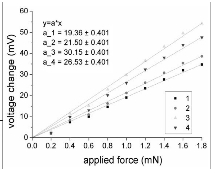
3. ábra Az érzékelők merőleges irányú terhelésre adott lineáris válasza
