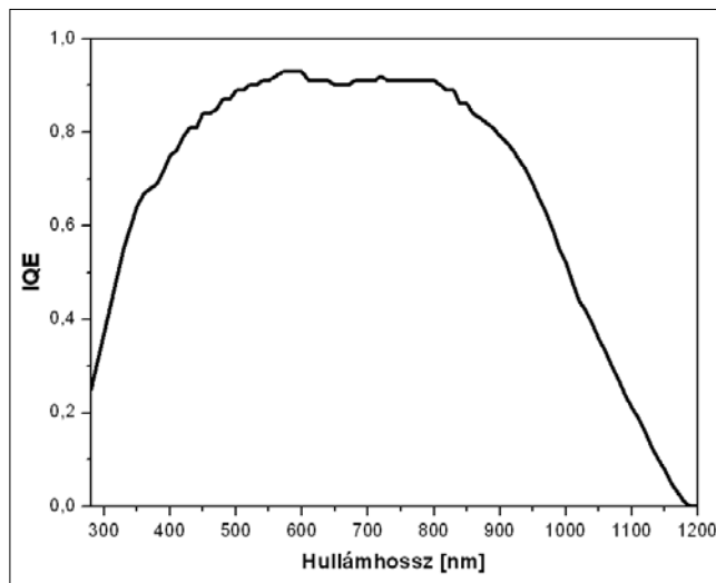
1. ábra PIII napelem jellegzetes belső kvantumhatásfoka
