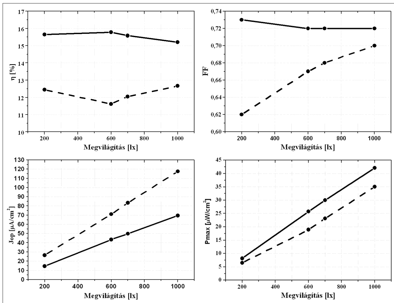
5. ábra Beltéri napelemek paraméterei különböző erősségű fluoreszcens beltéri megvilágítás esetében: hatásfok ( \eta ), kitöltési tényező (FF), maximális teljesítmény ( P_{\max} ) és a hozzá tartozó áramsűrűség ( J_{\text{op}} ) JB55 PIII cellára (szaggatott) és a-Si referencia cellára (folytonos).
