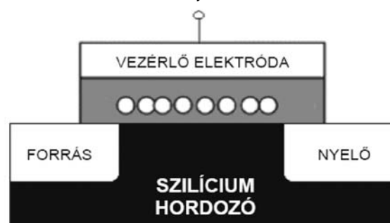
3. ábra A nanokristályos memóriatranzisztor
