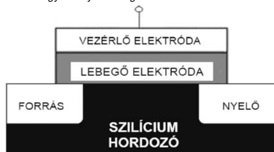
1. ábra Hagományos lebegő elektródás memóriatranzisztor
