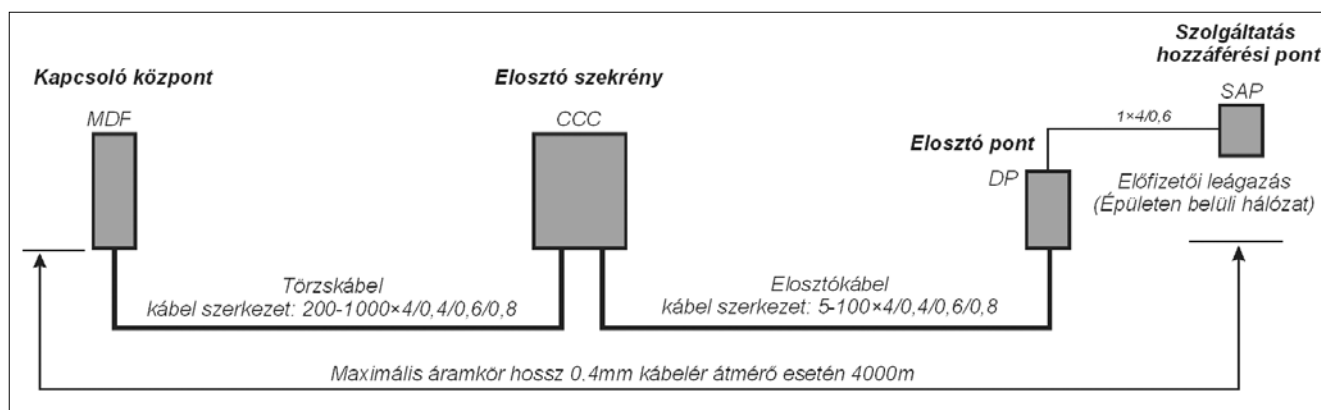
3. ábra A sodrott rézerű elérési hálózat felépítése
