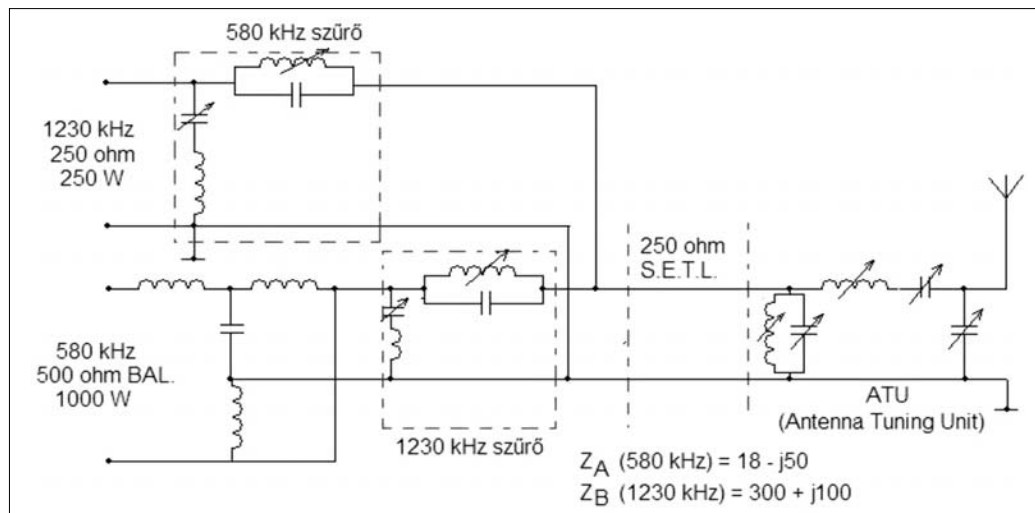
7. ábra Közép-angliai állomás diplexere
