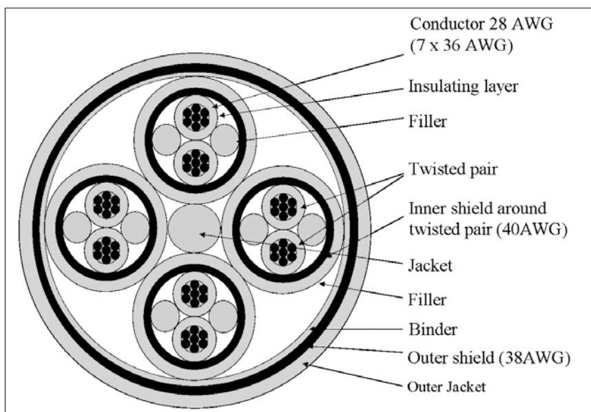
3. ábra A SpaceWire kábel
