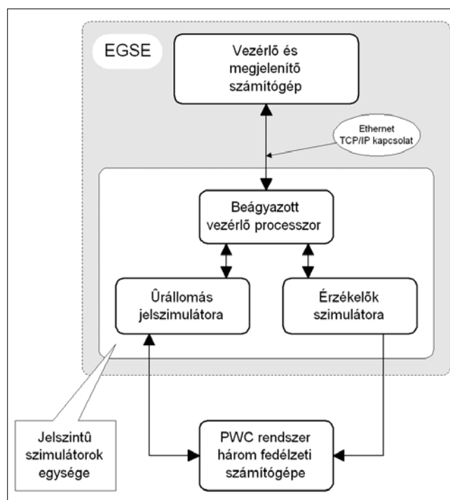
1. ábra A PWC EGSE rendszerének vázlata
