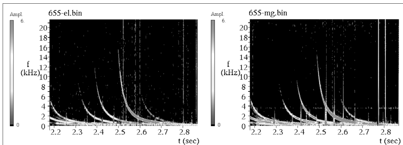
6. ábra A SAS2-K2 első mérési adatai, egy rendkívül erős whistler csoport elektromos és mágneses komponenseinek FFT képe, 2006. november 29., 5.00.00 UT Indonézia fölött
