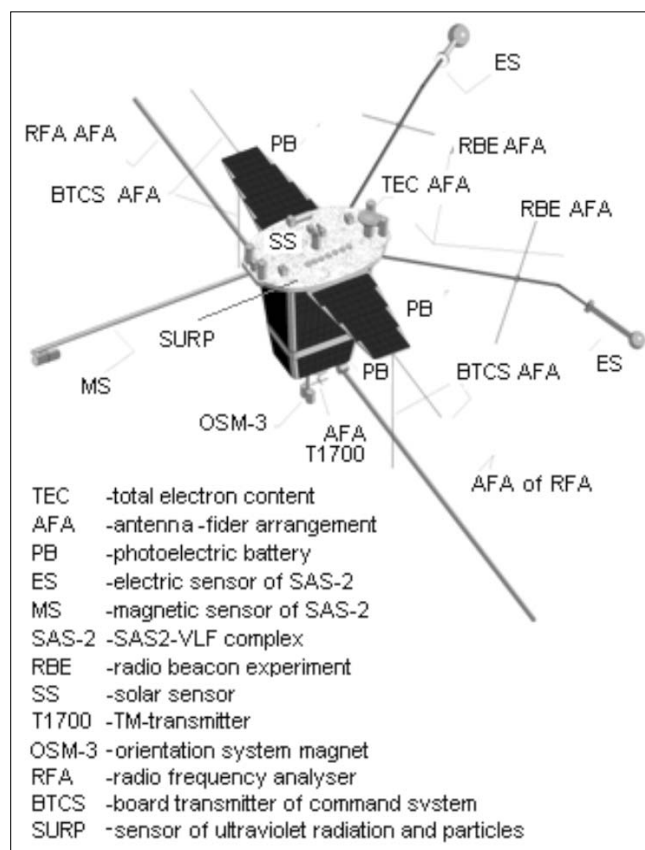
2. ábra A Kompas-2 vázlatrajza a műszerekkel. A SAS2-K2 érzékelői az ukrán gyártmányú két ES elektromos érzékelő és a szintén ukrán gyártmányú MS mágneses érzékelő.
