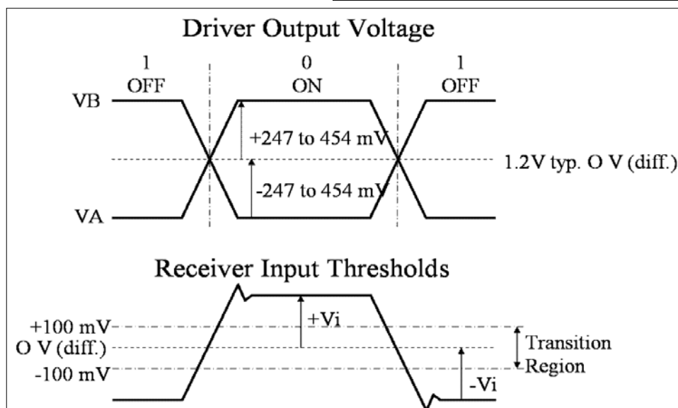
4. ábra LVDS jelszintek
