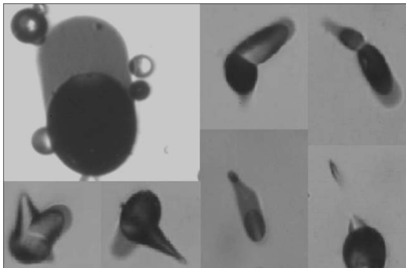
2. ábra Egy HZE, feltehetően a detektorban éppen leálló Fe részecske nyoma látható a bal felső sarokban, körülveve néhány fragmentum vagy meglökött mag nyomaival. A többi kép nagyenergiás neutronok által keltett magreakciók mikroszkópos felvétele a PADC nyomdetektorok felületén. A reakcióban keletkező részecskéket felismerhetjük arról, hogy nyomaik egy centrális pontból, az ütközés helyéről, különböző irányokba indulnak ki és hosszuk, illetve átmérőjük a keletkezett részecskék energiájától és rendszámától függ.
