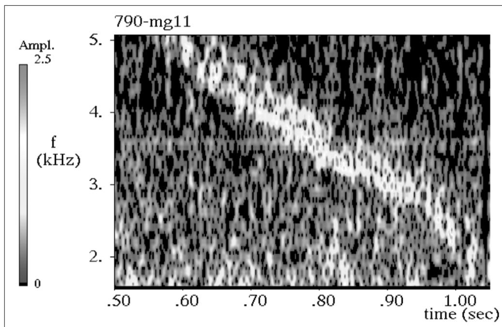
13. ábra A vezetett módusban terjedő whistler végső szakaszának FFT képe
