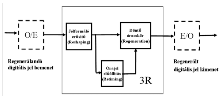
1. ábra Az elektronikus jelregenerátorok funkcionális felépítése
