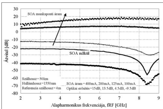
13. ábra Mért rádiófrekvenciás átvitel (a back-to-back optikai átvitelre normalizálva), különböző SOA munkapontoknál
