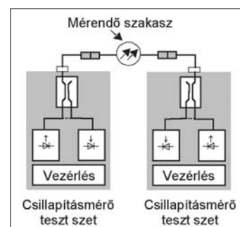
5. ábra Kétirányú csillapításmérés automatikus teszttel
