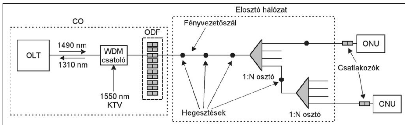
3. ábra PON hálózat sematikus felépítése
