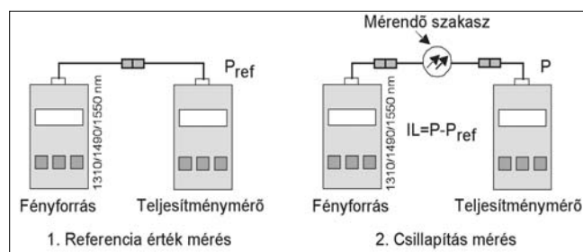
4. ábra Csillapításmérés fényforrással és teljesítménymérővel
