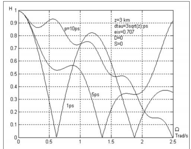
3. ábra AM átviteli karakterisztika Magyarázatot ad arra a paradoxonra, hogy a PSP gyorsabb elfordulása (nagyobb p ) miért okoz sávzélesség-növekedést. A nagyobb p az \Omega p/2 argumentumú trigonometrikus függvények szaporább változását okozza, ami szuperponálódik a futási idő különbség által létrehozott „állóhullám” görbére, megakadályozva annak zérusra csökkenését ( w=100 Grad/s).
