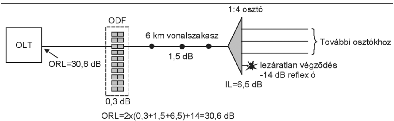
7. ábra Reflexió egy szabadon hagyott osztó kimenetről
