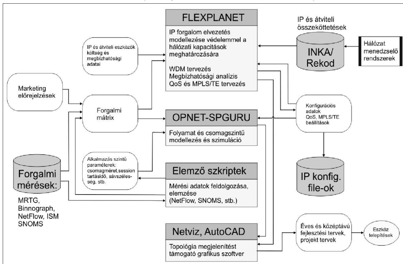
4. ábra Az NGN transzportrétegének fő tervezési elemei és adatbázis-kapcsolata
