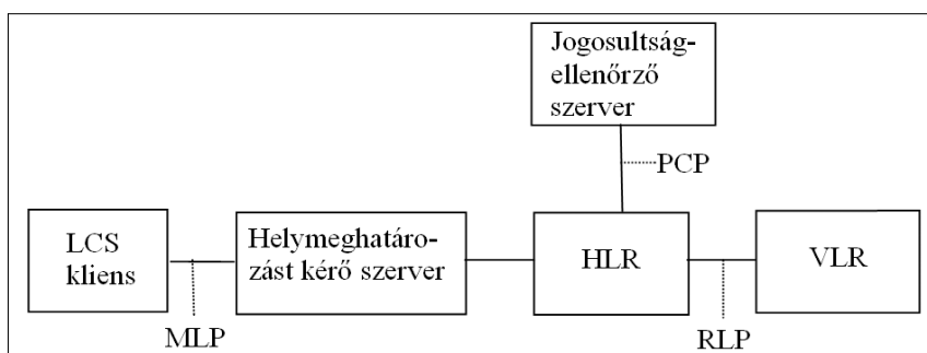
9. ábra A helyzetalapú szolgáltatások folyamatait tartalmazó MLS architektúra. Az MLP (Mobile Location Protocol) szerint lép kapcsolatba az LCS kliens a helymeghatározást kérő szerverrel, az RLP (Roaming Location Protocol) lép működésbe, ha az előfizető elbarangolt más hálózatrészbe, és a PCP (Privacy Check Protocol) ellenőrzi a kérés jogosságát.
