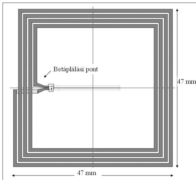
16. ábra Keretantenna nyomtatási képe 13,56 MHz frekvenciára
