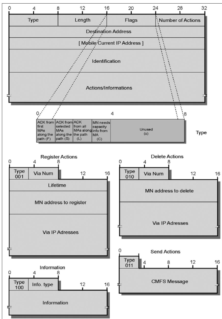
2. ábra A CMFSP üzenetstruktúrája
