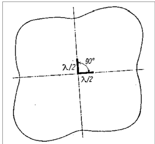
4. ábra HQ 1/0,4 típusú antenna horizontális karakterisztikája
