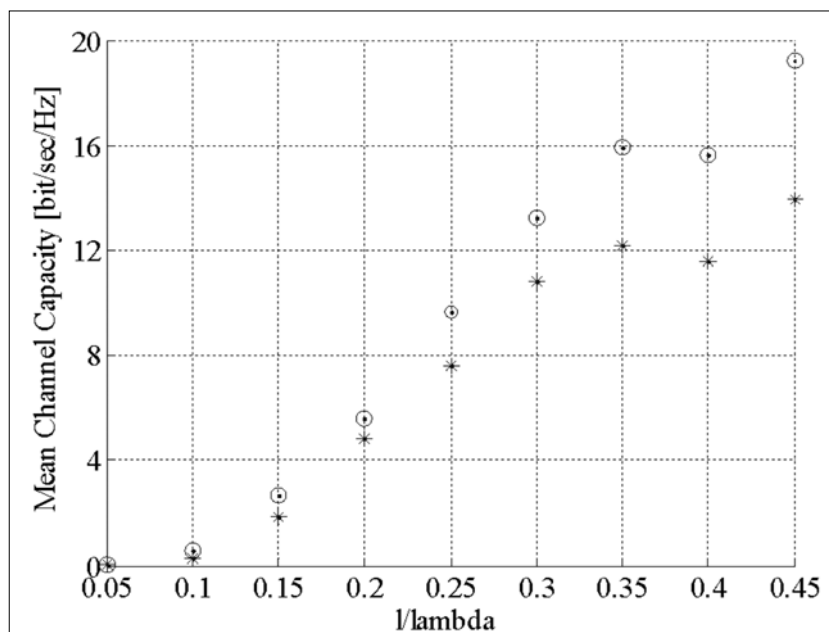
4. ábra 3x3 MIMO dipólantenna-rendszer csatornakapacitásának változása l/\lambda függvényében illesztett (o), illesztetlen esetre (*)
