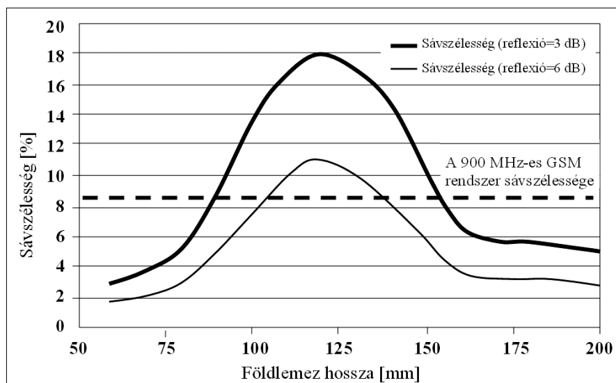
13. ábra PIFA antenna sávzélessége a földlemez hosszúságának függvényében
