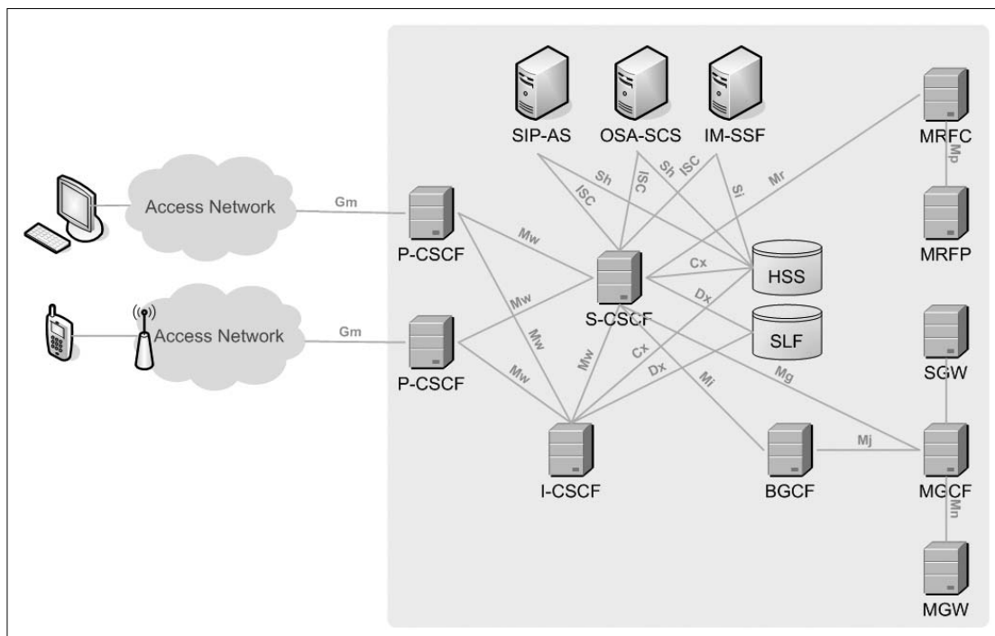
3. ábra IMS architektúra
