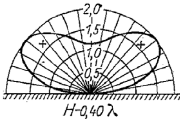
3/a. ábra HQ 1/0,4 antenna vertikális karakterisztikája
