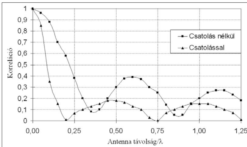
22. ábra Vevőantenna vételi jelének korrelációja az antennatávolság függvényében Rayleigh-fadings csatornára
