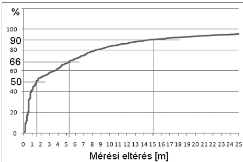
6. ábra Kültéren elvégzett mérés eredményei, azaz hány százalékban volt a mérési pontosság az adott távolság alatt.
