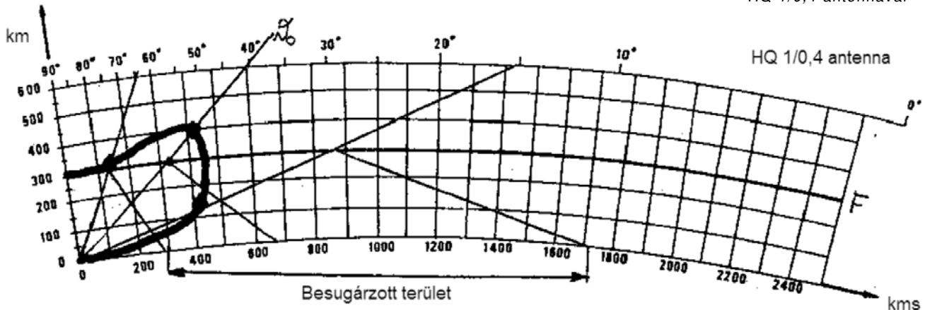
3/b. ábra Elérhető sugárzási terület nagysága egyugrásos átvitel esetén HQ 1/0,4 antennával
