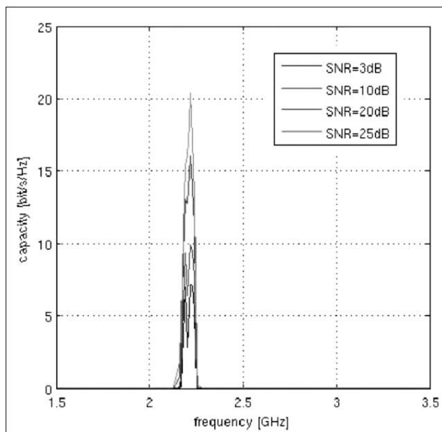
7. ábra Számított csatornakapacitás-értékek a frekvencia függvényében – lapközép-antenna esetén
