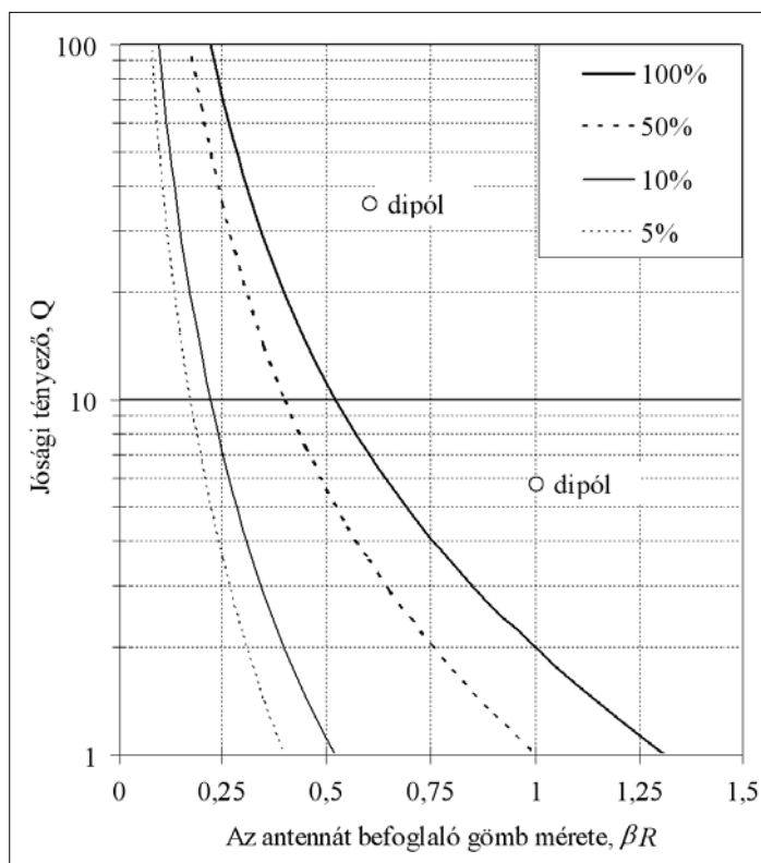
7. ábra Idealizált antenna minimális jósági tényezője az antenna hatásfokával paraméterezve
