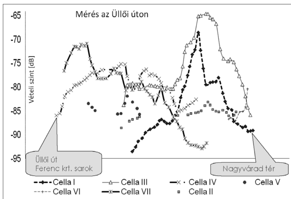
1. ábra GSM vételi viszonyok az Üllői út egy szakaszán. Megfigyelhető a bázisállomások vételi szintjének helyfüggősége, amely a helymeghatározást lehetővé teszi.
