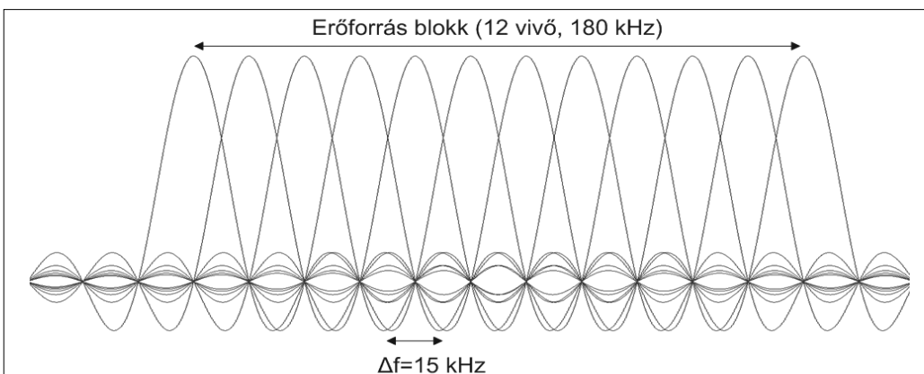
6. ábra Erőforrás-blokk frekvenciatartománybeli felépítése
