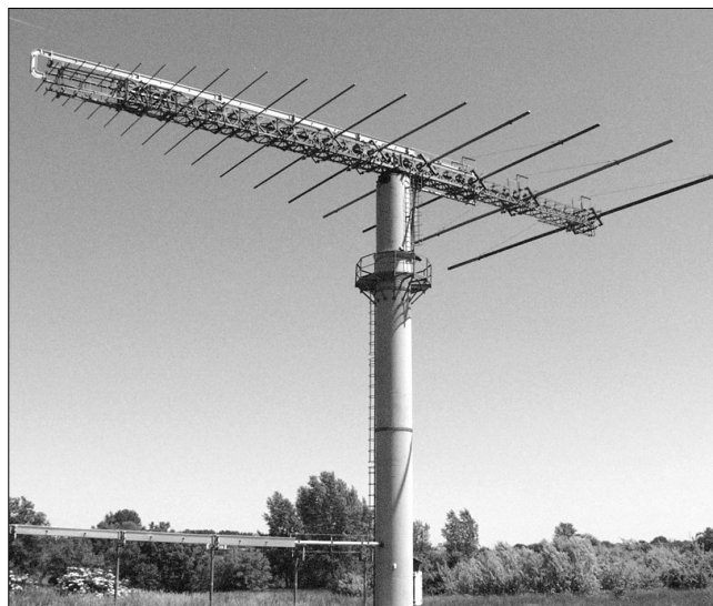
5. ábra Thomcast gyártmányú log-per antenna
