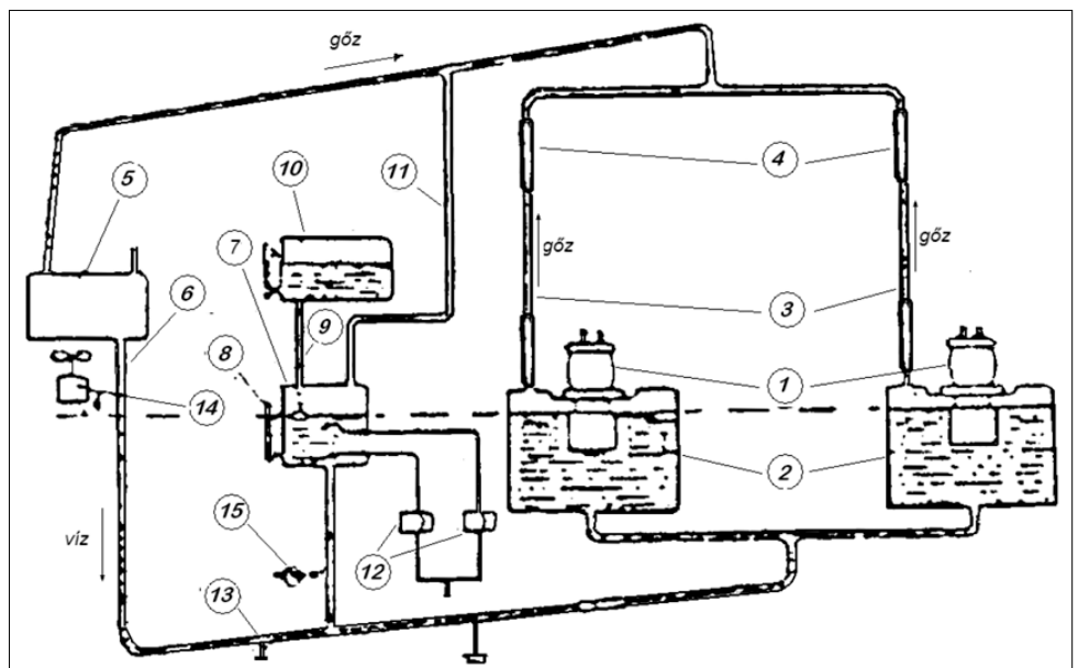
8. ábra Az elgőzölögtetési alapú hűtési rendszer
