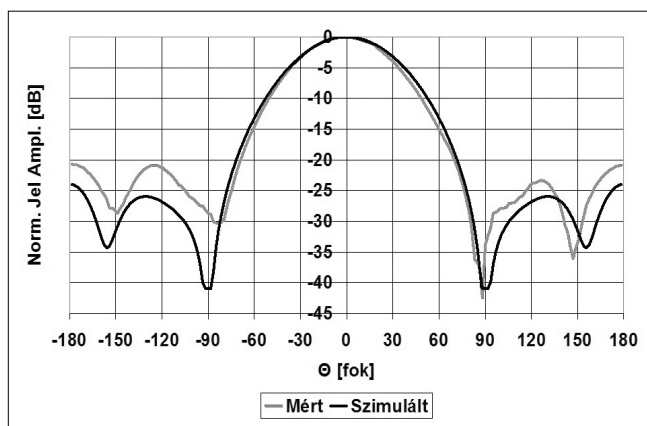
15. ábra E síkú biquad iránydiagramok
