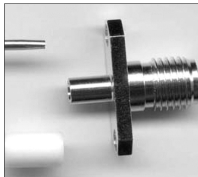
8-9. ábra A használt csatlakozó és az elvégzett forrasztás
