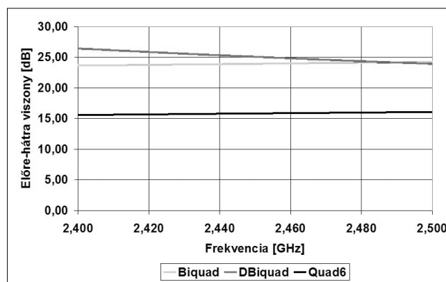
4. ábra Szimulált előre-hátra viszonyok
