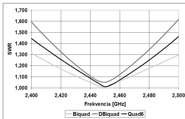
2. ábra Szimulált állóhullámarányok
