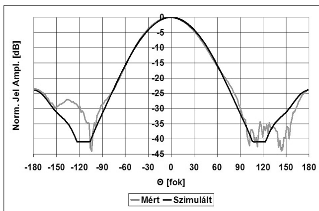
18. ábra H síkú biquad iránydiagramok
