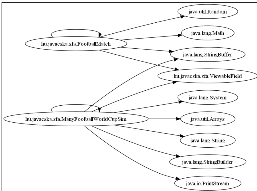
1. ábra Nem az indítástól, hanem a 250000. metódushívástól további 17 millió hívás alapján készített gráf
