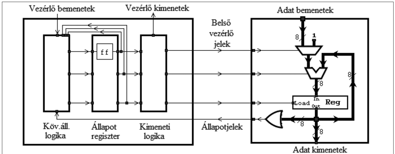
1. ábra Mikroprocesszor jellegű rendszerek általános modellje
