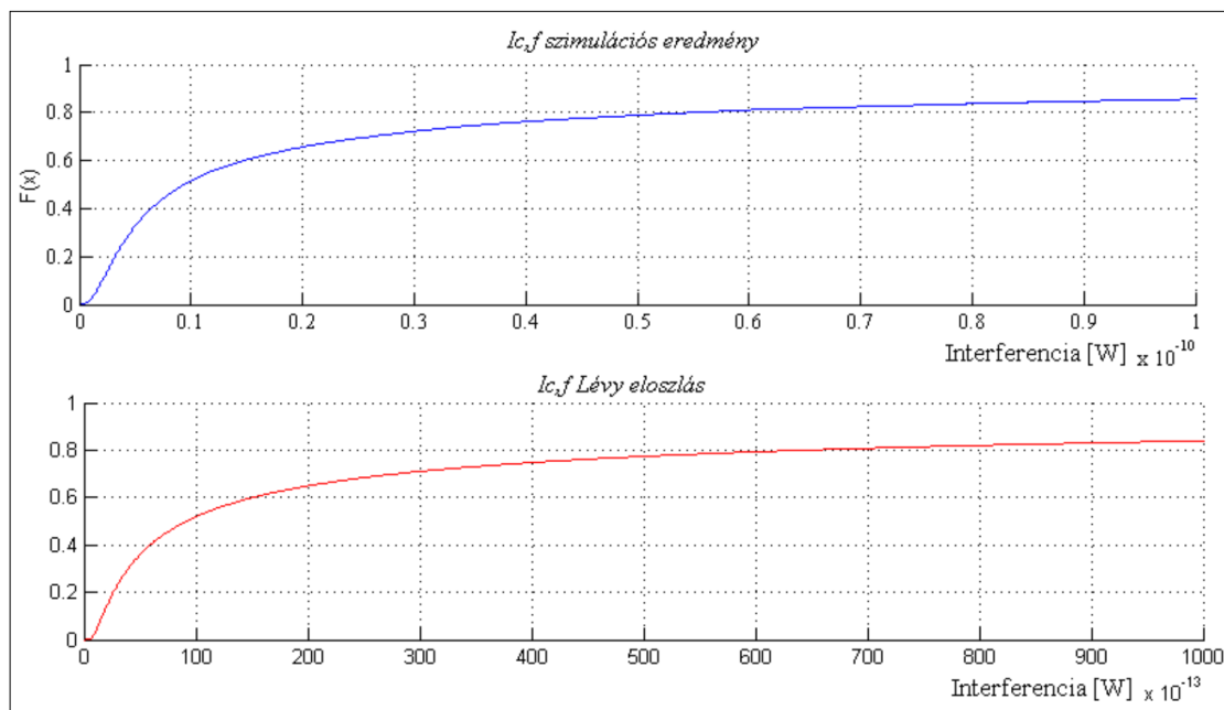
8. ábra Lévy-eloszlás igazolása makro-femto interferencia esetében (belváros)
