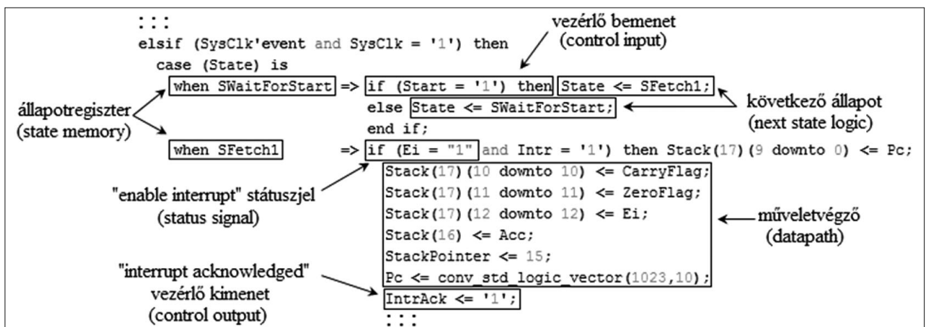
2. ábra Egy egyszerű mikroprocesszor FSM típusú VHDL modelljének részlete
