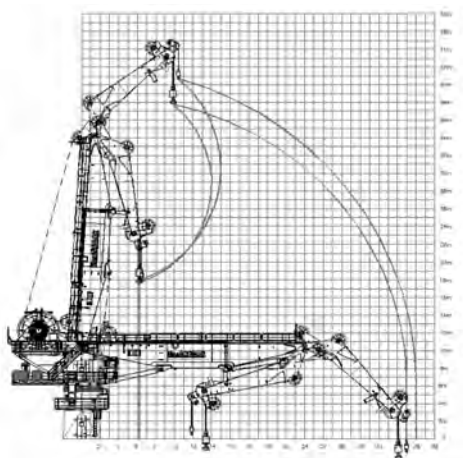
6. ábra. Daru emelési mechanizmusa (working area diagram)
