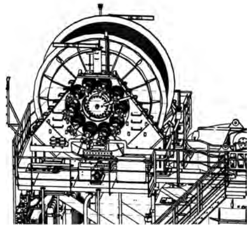
5. ábra. Offshore AHC winch
