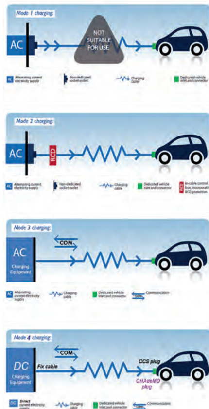
3. ábra: A szabványokban meghatározott töltési módok
