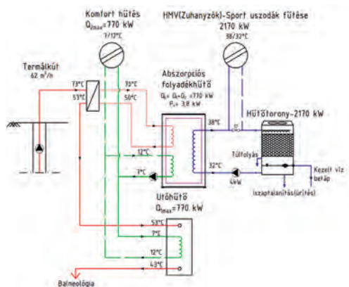
1. ábra: A termálvizes hűtőrendszer egyszerűsített kapcsolása
