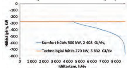
2. ábra: A vizsgált rendszer hűtésitartam-diagramja
