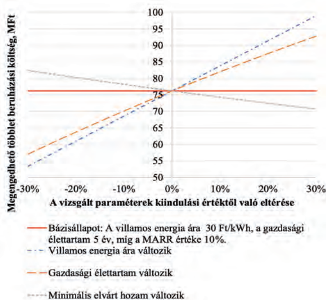
4. ábra: A megengedhető beruházási többletköltség érzékenysége a meghatározó paraméterek változására
