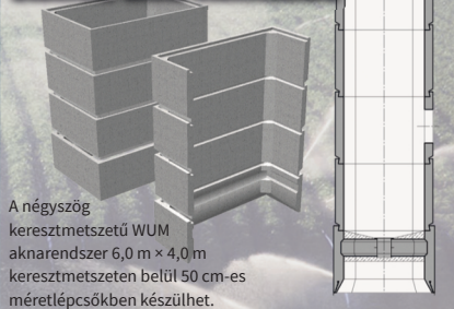
WUM négyyszögletes vasbeton átemelő akna elemcsalád
