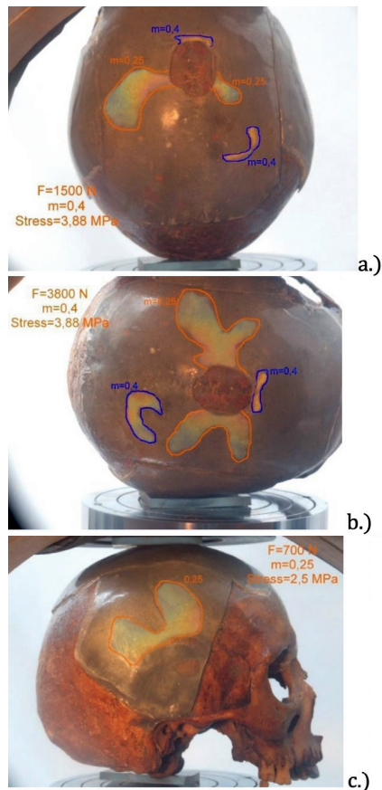
7. ábra Koponya határterhelésének megállapítása érdekében végzett vizsgálatok – a) koponya előlől terhelve, b) koponya oldalról terhelve, c) koponya felülről terhelve [6]
