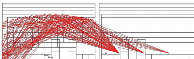
4. ábra A Bánffy terem nézőtérben lévő hangvetők vizsgálata (Alabárdos Zsuzsanna, Arató Akusztikai Kft.)
