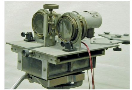
4. ábra Szórt fényű reflexiós polarizskóp (Nagy-Szittner-féle) [3]
