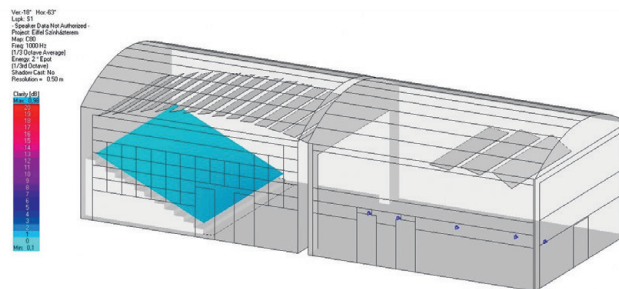
3. ábra A Bánffy terem számított hangtiszta fokoka 1000 Hz – 1/3 októvában (Alabárdos Zsuzsanna, Arató Akusztikai Kft.)
