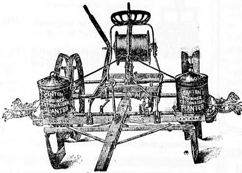
„SENIOR“ tengeri űltetőgép autom. négyzet űltetőkészülékkel.
