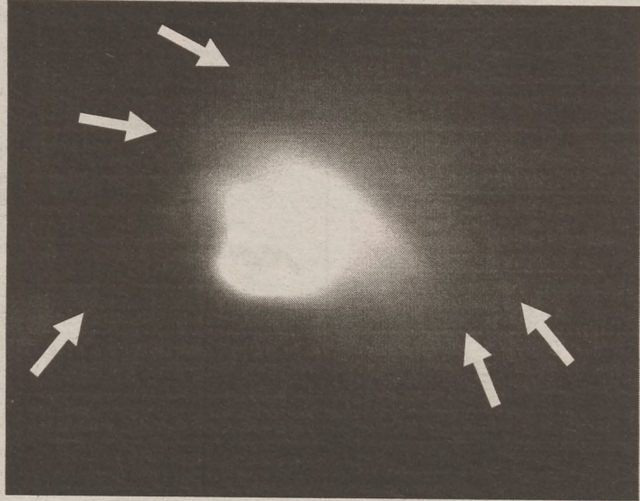
Borkovits Tamás (BKkM-i Önk. Csill. Int. Baja) CCD képe a Hale-Bopp üstökös magjának közvetlen környezetéről (50 cm f/8,4 RC)
