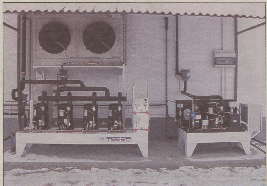
Az üzem teljes melegvízszükségletét a csoportosítottággal hulladék hője biztosítja
