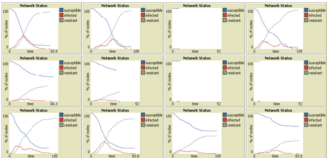
2. ábra: Járványgörbék a Vírus a hálózaton modellben (Stonedahl–Wilensky 2008 alapján).
