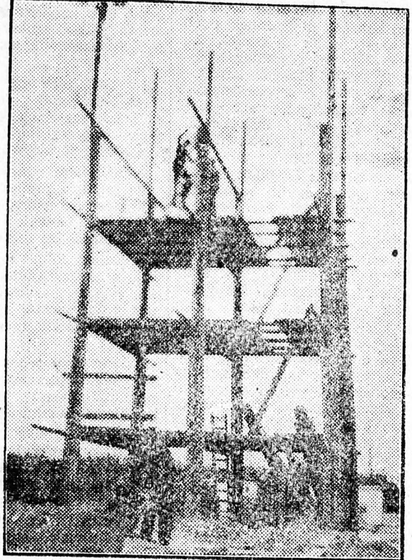
A 15 méteres torony állványzata
