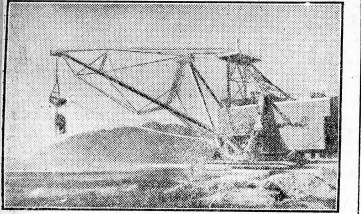
Hatalmas ütemben folyik a Volga-doni hajózható csatorna építése. A munkálatok gyorsan haladnak előre: hírszén a legfejlettebb technikát használják fel a nagyarányú építkezéshez. A képtünkön az urai gyárban készített hatalmas exkavátort látjuk munka közben.
