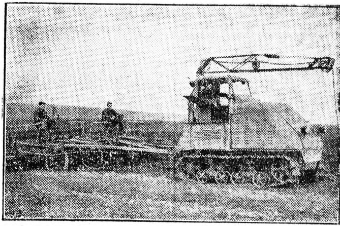
Az Ukrán Szovjet Szocialista Köztársaság korszerű—seveszkövi gép- és traktorállomásán a tavaszi munkák során minden perccel kihasználják a 34,7 lóerős elektromos traktorokkal. Képeinken egy villany-traktort láthatunk földmunkálás közben
