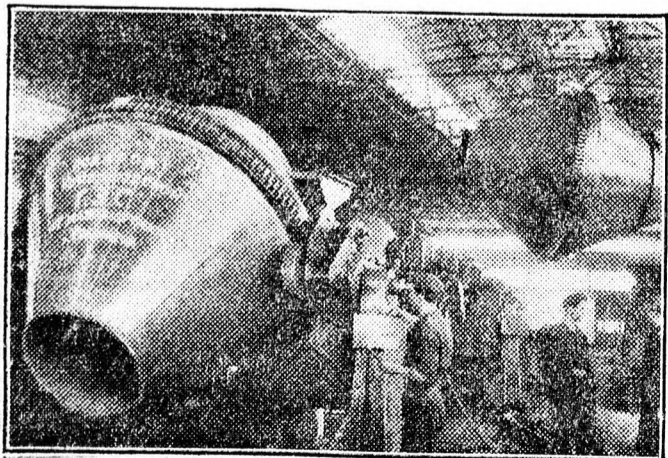
A képen látható 2100 és 4500 ürméretű betonkeverő őrlásgépeket a kujbisevi vízierőmű számára készítették a szlavjanszki építőipari gépgyárban
