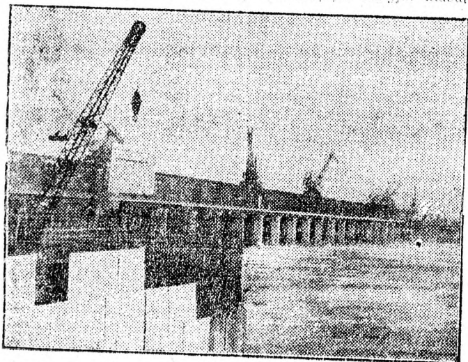
Befejezéséhez közeledik a hajózható Volga-Don csatorna egyik nagy építkezése, a címjanszkajai vízierőközpont. Képiünkön a szerelő betonozók a gát lámpáit ember nagyságú burkolólapokkal fedik.
