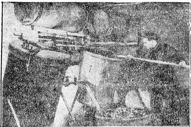
A „Vorosilov” kolhoz fejlett állattenyésztő telepén külön takarmánykocsikat létesítettek, ahol univerzális malom őrli meg a takarmánygabonát, felszelelteti a takarmánygyökereket, összezúzza az olajpogácsát. A képen M. Kurlajev kolhozparaszti tápláló takarmányt készít a takarmánykocsijában az állatok számára.
