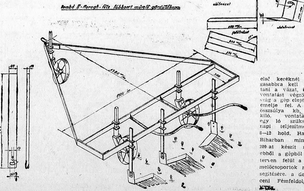
Szabó-Horváth-féle többsoros művelő gördülő kapa
