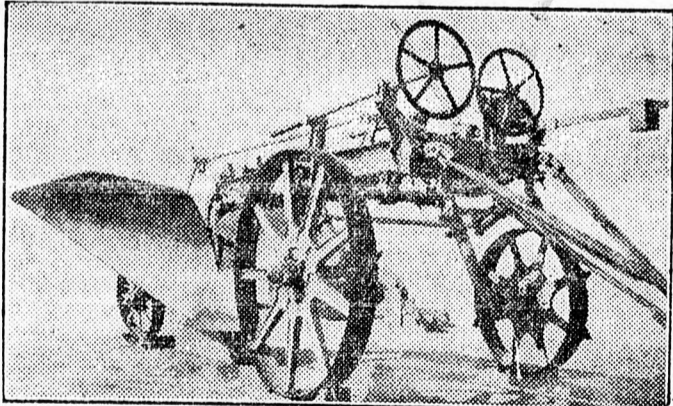
Új típusú traktorvontatású rigol. Eke szőlővényre és gyümölcs-facsemeték 60 centiméter mélyen történő elültetésére.
