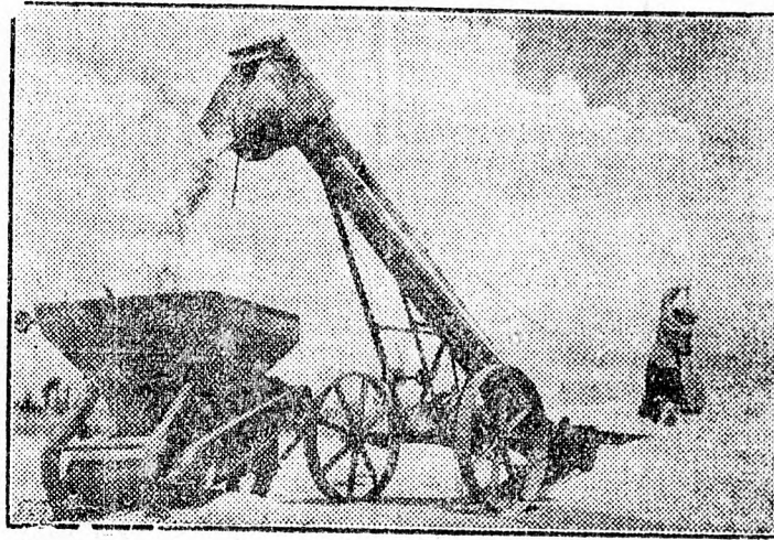
Egyre több helyen állítanak fel magaszórákat, amelyek óránként 10-12 tonna magot forgatnak meg és ezzel lehetővé teszik a nedvességtartalom gyors csökkentését. Futószalagon ömlik a búza a folyópárti uszályokba, hogy víziúton is eljusson az idej gazdag aratás bő termése a begyűjtő állomásokra.
