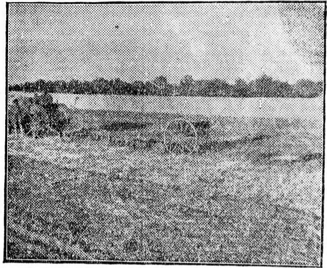
G. Nagy László, a szoboszlói géppállomás brigádvezetőjének gépkapcsolási újítása egyszerre négy művelet végzésével gyorsítja a másodvetést.
