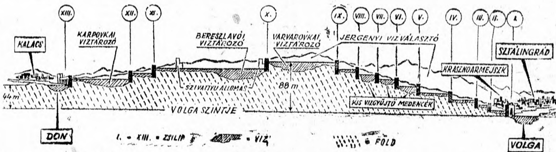
A Volga—Don közének és a nagy csatorna útvonalának hosszanti keresztmetszete.
