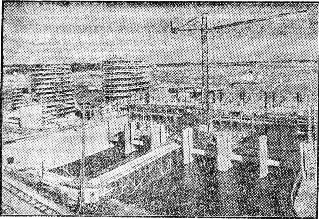
Épül a tiszalöki vízierőmű.
