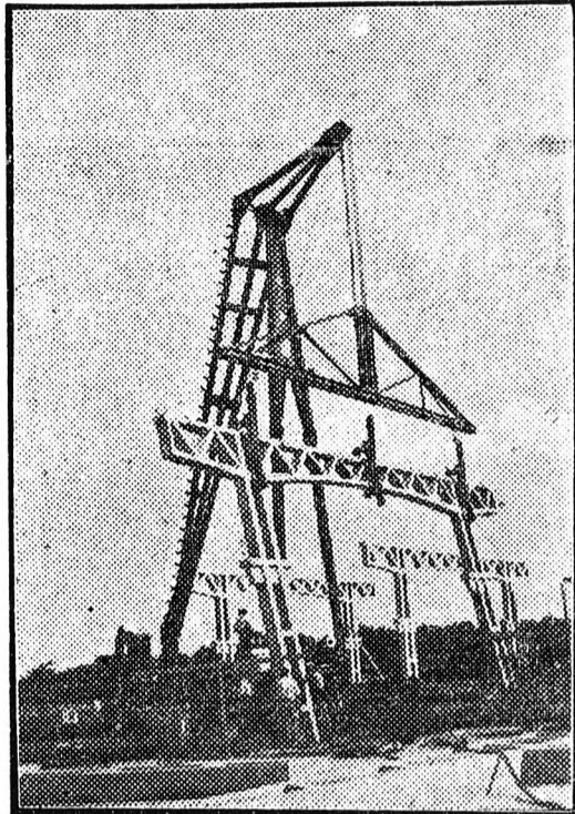
A napokban kezdtek meg a 15 ezer négyzetméter alapterületű tizenegy hajós nagy csarnok vasbeton kerettartóinak beemelését. Képiükön a 18 tonnás Szűke-daru beemeli a földön előre elkészített beton kerettartót.
