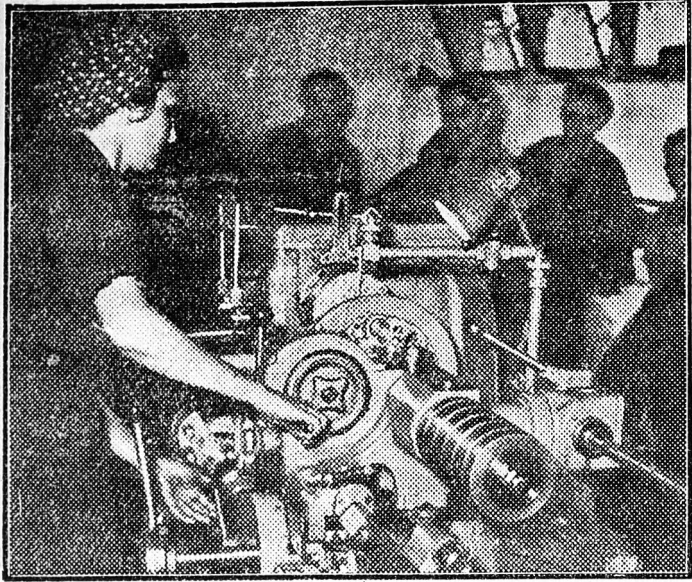
Nagyteljesítményű szovjet gyártmányú gépek segítik a Golyósesapágygyár átképzés üzemének munkáját. A képen az M. 1336. számú R-17-es típusú szovjet esztergagép látható, melyen Szarvas Ilona ifjúmunkás dolgozik. Jelenleg belső gyűrűt készít. Havi átlagteljesítménye 150 százalék.
