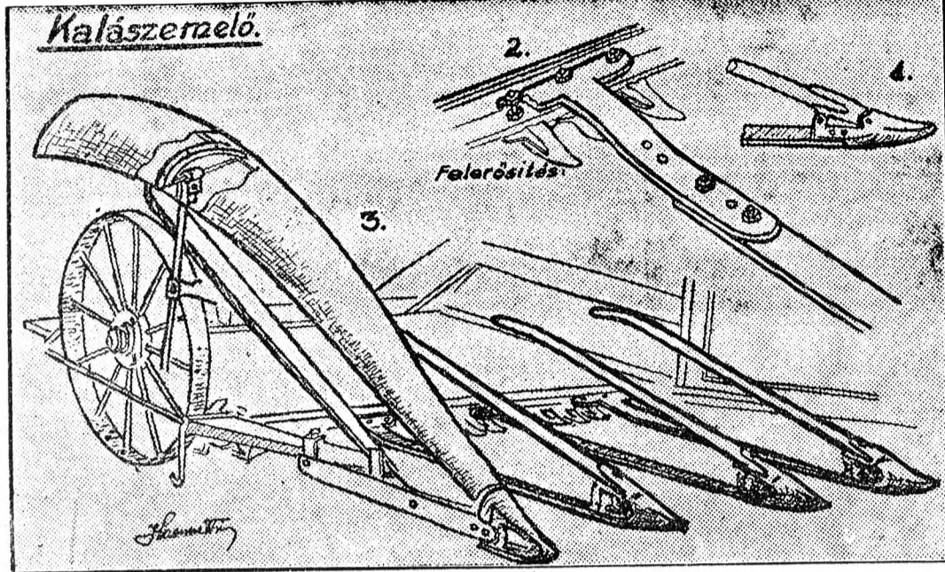
Az aratás gyorsítása, a dült gabonánál megköveteli, hogy a szempergés elkerülése érdekében az aratógépeket minél előbb szereljék fel kalászemelővel. A képen a kalászemelő (I), a felerősítés módja (II.) és az összeszerelés (III.)
