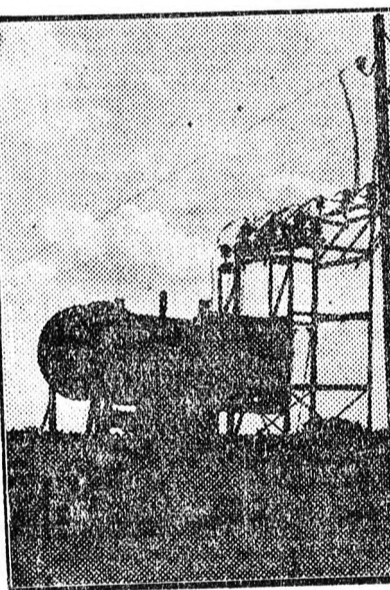
A mozgó transzformátor bekapcsolása a hálózatba.
