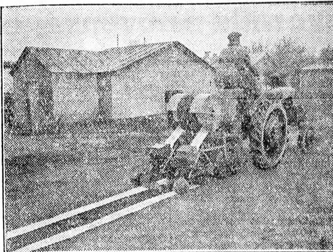
A képen: a kétsoros felfüggesztett vetőgép kipróbálása a moszkvai K. A. Tyimirjazov Mezőgazdasági Akadémia kísérleti zöld-ségtermelő gazdaságában. — Fotó: V. Sarovszkij.
