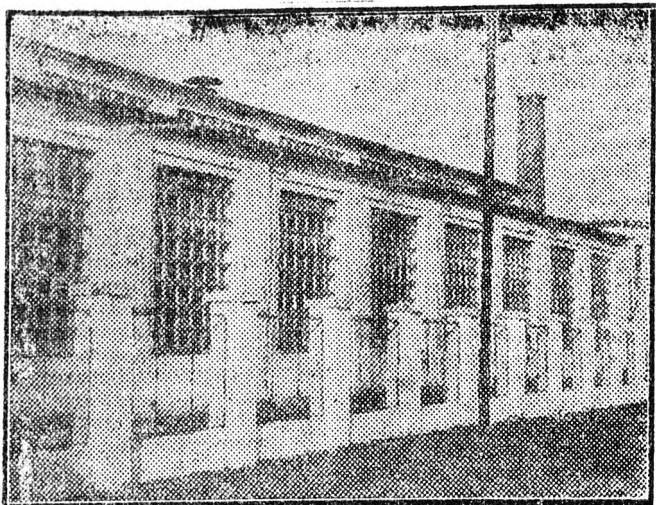
Tegnap avatták fel az öt éves terv országos viszonylatban is jelentős létesítményét, a Hajdú megyei Lakatos és Gépipari Vállalat új üzemét. Képünkön az öntőde épülete.
