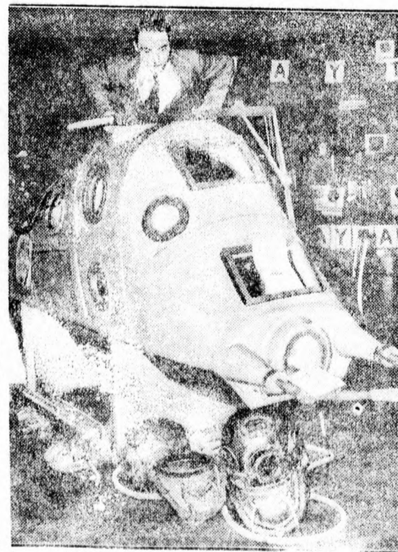
Egyszemélyes buvárhajó
