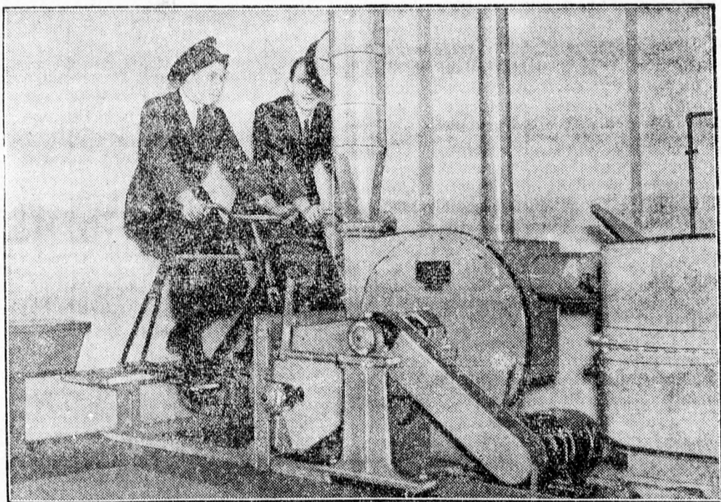
London nagy bankjai is megépítették a légvédelmi pincéiket s egyes helyeken a szellőztető készüléket bicikliszerű pedálhajtásra szerelték. Képünk egy ilyen szellőztető készüléket ábrázol
