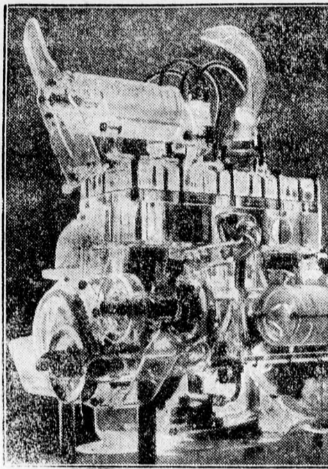
A berlini gépkocsikiállításán látható egy szemelelykocsij teljes gépezete, amely teljesen átlátszó anyagból készült, hogy működés közben ellenőrizni lehessen a legapróbb kerék fordulását is.
