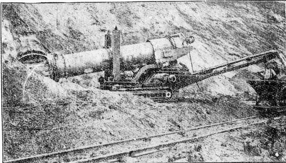
Új rendszerű aknafuró, amelynek főleg a szén-, vagy kőbányákban veszik nagy hasznát. A készülék gömbölyű feje a kifurt föld, illetve kő-rőlősiéget hátravetve annak elszállítása aztán igen könnyen megtörténhetik
