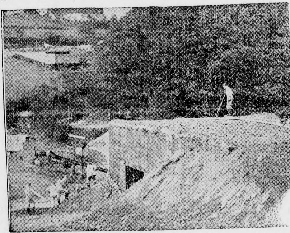
Németország nyugati határerődítéseiről ezek az első fényképfelvételek. Első képünkön az egyik határerődítés építése, másik képünkön a tankelhárító vasbetonból készült akadályok láthatók
