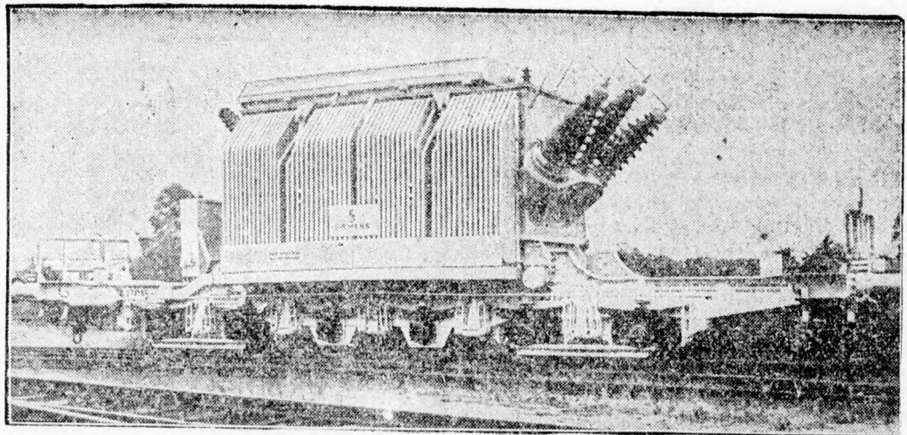
A Siemens művek új, 120.000 waltos hatalmas mozgó transzformátort készítettek Svédország számára. A transzformátor alváza kerekeken jár, úgy, hogy bárhova szállítható európai vasuti síneken, ahol hirtelen nagyobb áramfogyasztásra van szükség.
