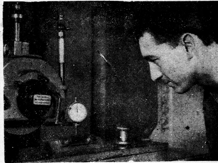
Korszerű sikközörögépet szerzett be az üzem az NDK-ból. A gépen Báthori Lajos lakatos beállítja a munkadarabot az elektromágneses asztalra és a beállítás pontosságát ellenőrző órával biztosítja.
