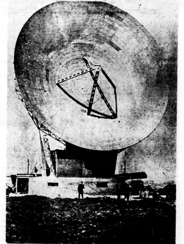
A július 10-én kilőtt Telstar mintájú amerikai mesterséges holdnak, amely televíziós adások és telefonbeszélgetések továbbítására szolgál, angliai óriás antennája Goonhilly Downs-ban van. A képen: a Goonhilly Downs 800 tonnás óriás antennája
