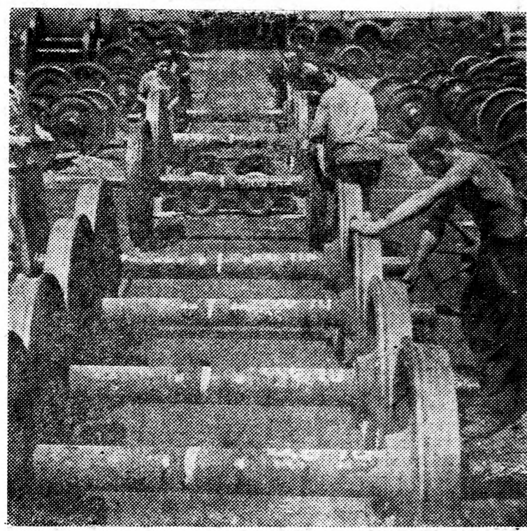
A járműjavító kerékosztályában naponta 50 pár vasúti vagonkerék felújítását végzik el. Ezenkívül havonta 20 darab komplett mozdonykerék garnitúrát javítanak fel. Képünkön a Fazekas brigád elszállításhoz készíti elő a felújított vasúti vagonkerékeket
