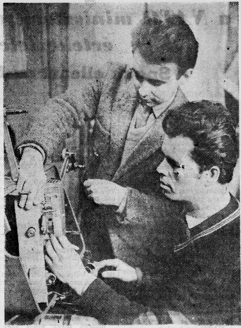
A Hajdú-Bihar megyei Moziüzemi Vállalat műszaki műhelye gondoskodik a filmszínházak zavartalan üzemeléséről. Havonta egyszer a megye és Debrecen minden moziját ellenőrzik és a hibás gépeket azonnal javítják. Havonta mintegy 40—50 vetítőgépet és erősítő berendezést vizsgálnak át. Képviselet Erdős László műszerész és Papp Béla rádióműszerész 16 mm-es vetítőberendezést szerel össze
