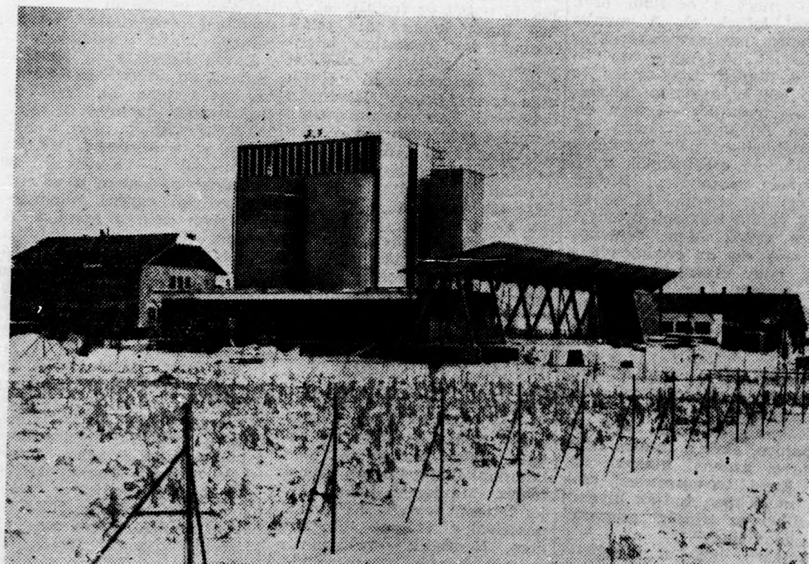
A nemesgulácsi új ásványvíz miben megkezdődött a gépek próbajáratása. Ezen te nyolcezer tonna hegykréta- és okker-alapanyagot zúznak az örlőmüben. Ezzel a mennyiséggel kiegészítik a hazai festék- és vegyipari gyárak igényeit. A hegykréta-alapanyagot az örlőmüben 15 kilométerre a Hegyesdől, az okker-alapanyagot pedig 30 kilométer távolságból, Cserszegtomajról szállítják gépkocsikkal. Az új ásványvíz március végén kezdi meg a termelést. Képünk az új ásványvíz művet ábrázolja (MTI Foto — Mező Sándor felv.)
