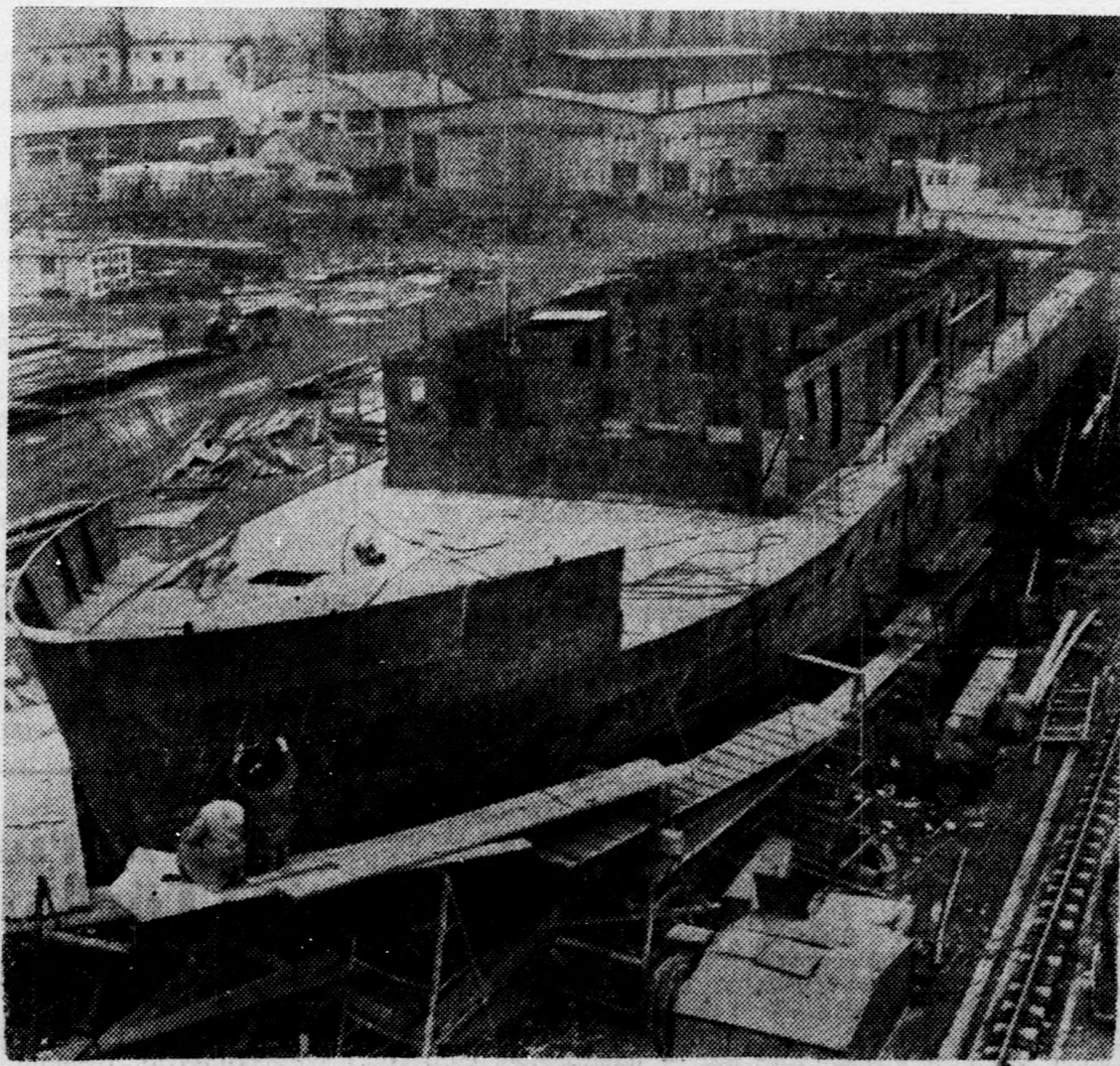
A felszabadulási munkaverseny során öt nappal, a határidő előtt befejezték a balatonfüredi hajógyárban épülő 1200 tonnás folyami vontatóhajó hegesztési munkálatait (MTI Foto — Kovács Sándor felv.)
