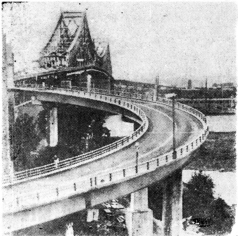
Kanadai híd, melynek burkolatát epoxigyantahabarcból készítették
