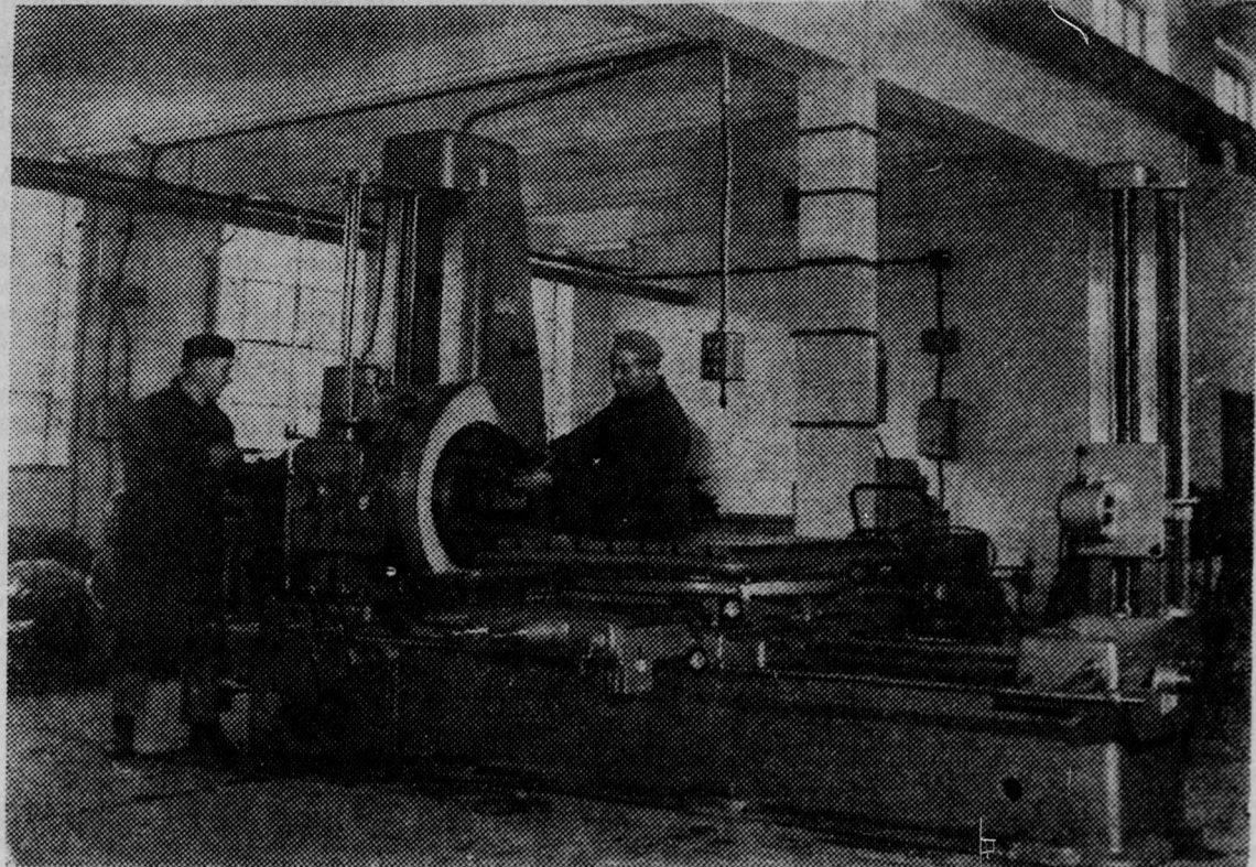
A ktsz egyik legdrágább munkagépe: a Horizontál típusú fűrőmaró mű, mely nagy segítséget nyújt majd a forgácsolási műveletekhez. Képünkön a 400 000 forintos gép beállítását végzik a szerelők az új üzem faiparigépgyártó csarnokában
