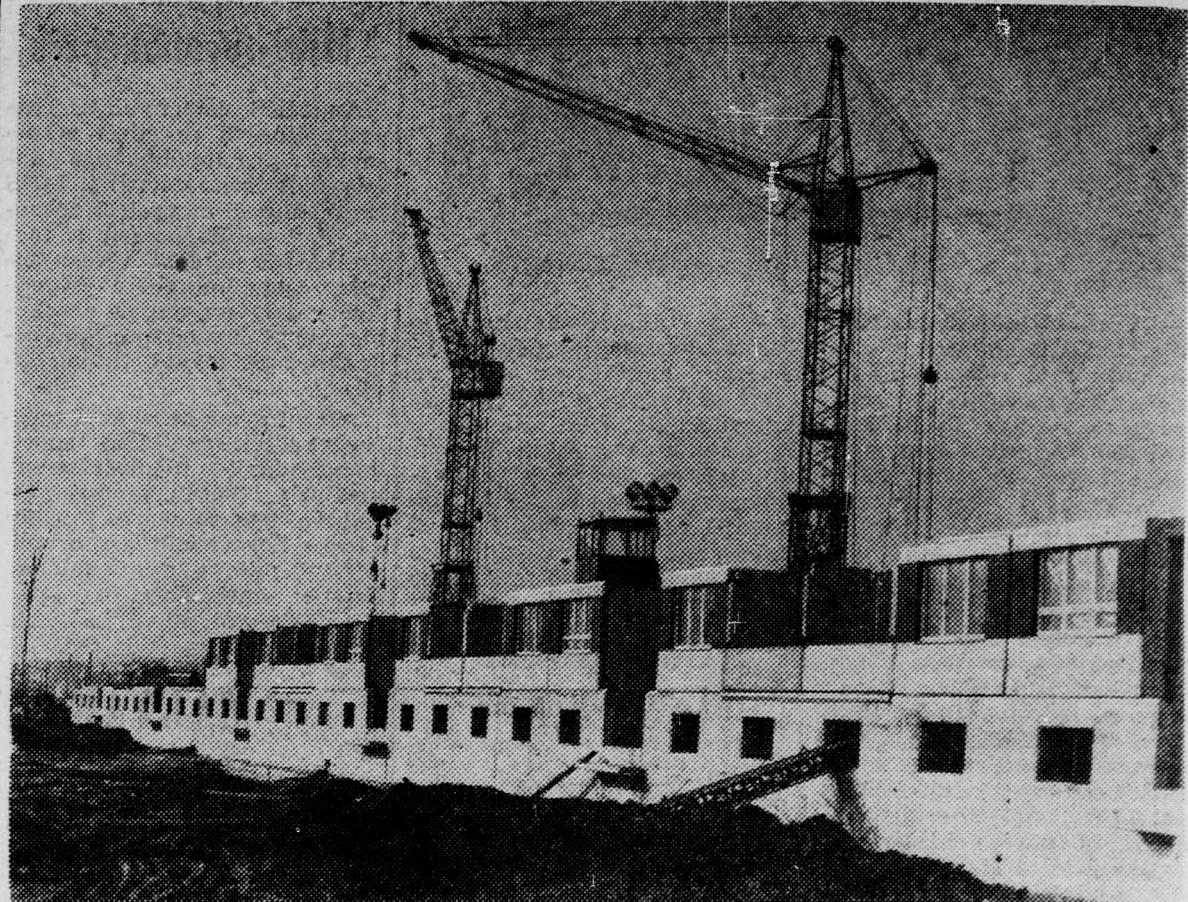
Hatalmas, speciális szállítókoszikkal érkeznek a helyszínre. Nagy teherbírású, szovjet toronydaruk emelik be a falakat. Alul jól láthatók a garázsablakok
