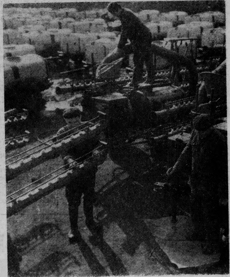
A Budapesti Mezőgazdasági gépgyár debreceni gyáregységében készül a RSHA nagynyomású ventilátoros permetezőgép, a Rapidtox szuper gépcsalád új tagját a moszkvai kiállításon mutatja be a gyár előzőr. Az új típusú permetezőgéphez sokféle kiegészítő gépegység tartozik. A képen: szállítás előtt ellenőrzik a gépeket (MTI Foto — Hadas felv.)
