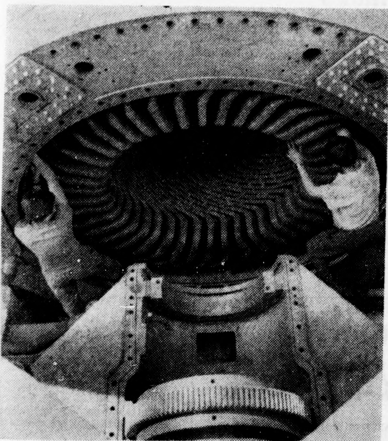
Nemsokára befejezik a második 150 megawattos turbina szerelését Százhalombattán. Az új gépegyes beindításával a Dunamenti Hőerőmű teljesítőképessége eléri majd a 440 megawattot. A képen: beállítják a 150 megawattos turbina állorészét
