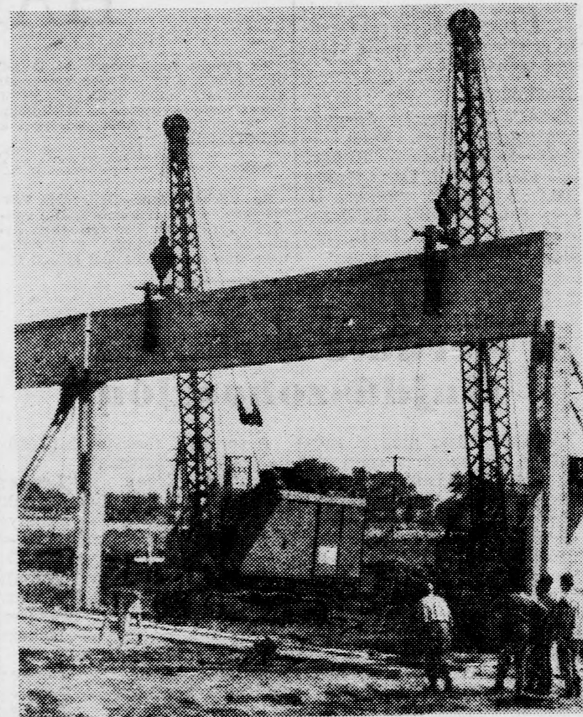
Nagy daruk segítik a főtartók beemelését. Egy-egy ilyen épületelem súlya: 18 tonna (Köszeghy György felv.)
